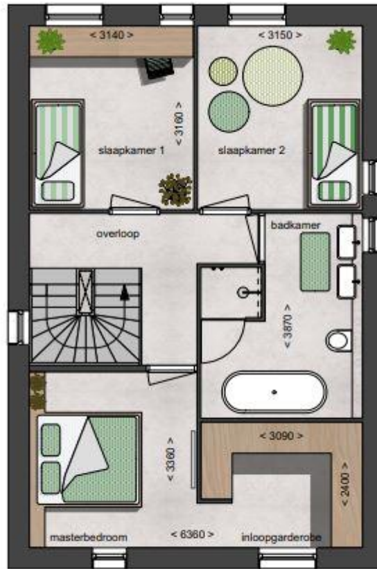
Eerste verdieping
